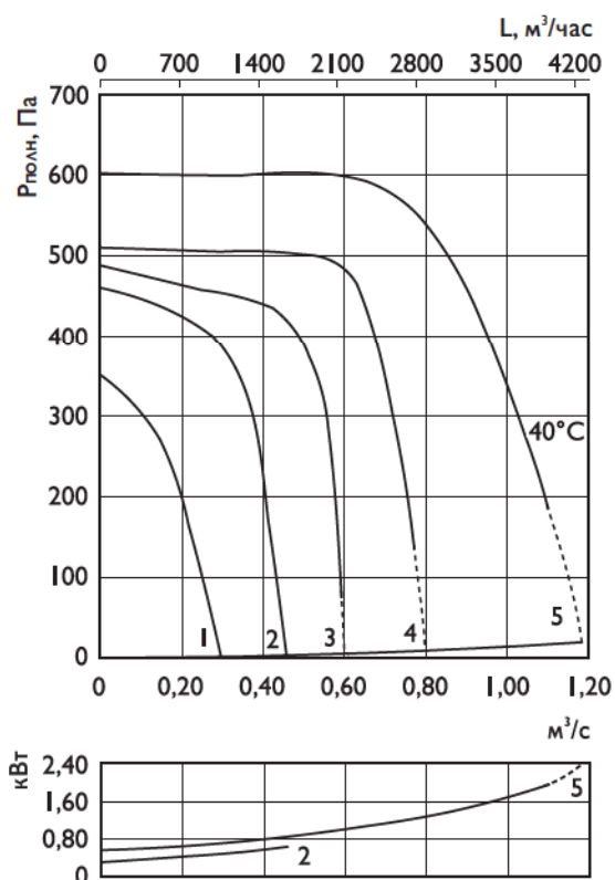
RK 600×350 E1/RKC 355 E1
