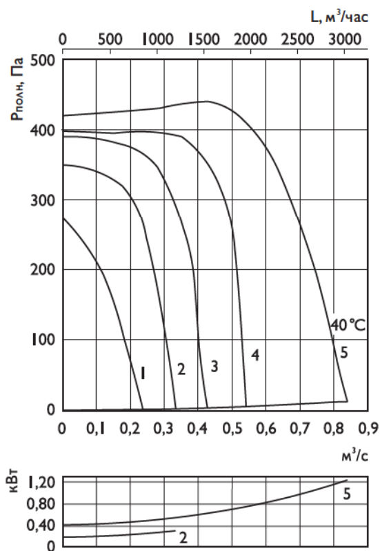
RK 600×300 F1/RKC 315 F1
