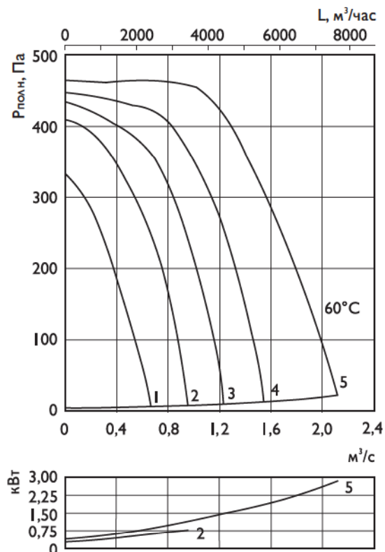
RK 800×500 E3/RKC 500 E3
