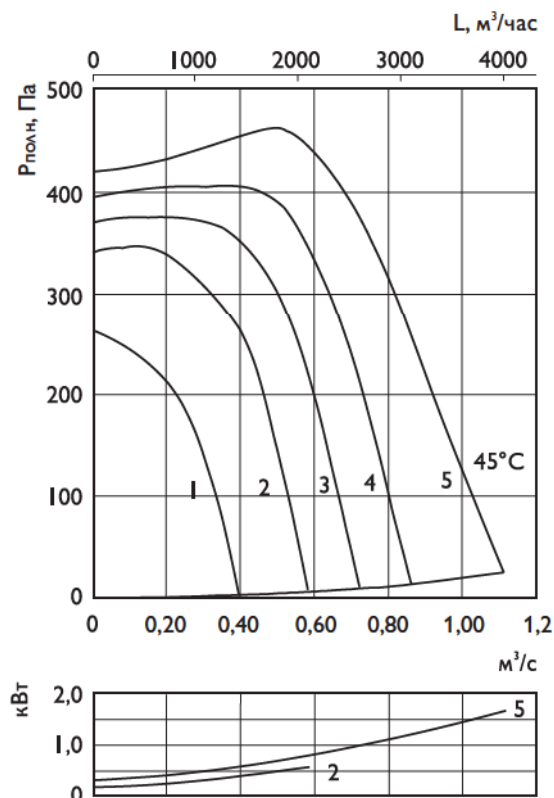
RK 600×300 F3/RKC 315 F3
