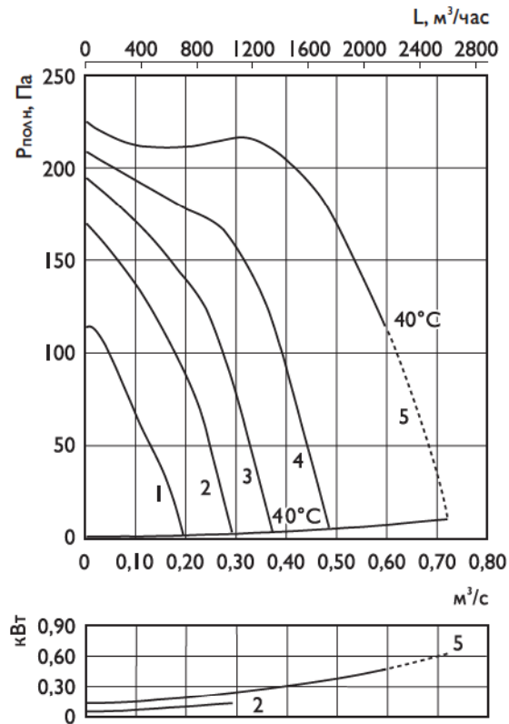
RK 600×300 D3/RKC 315 D3
